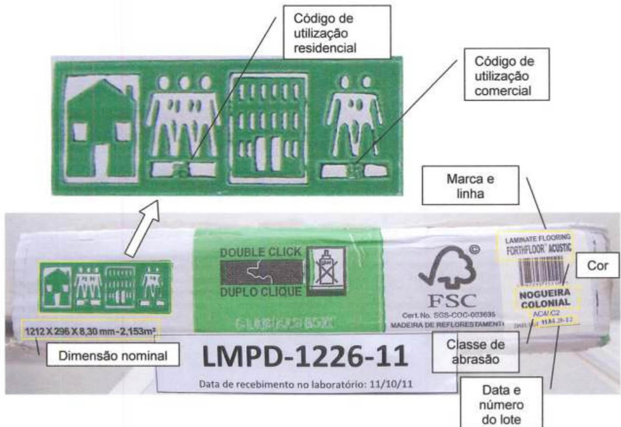
Fotos 2 e 3 – Informações impressas na embalagem da amostra recebida: códigos do sistema de classificação para categorias de utilização (detalhe ampliado), dimensão nominal, marca, linha, cor ou padrão, classe de abrasão, data e número do lote.
